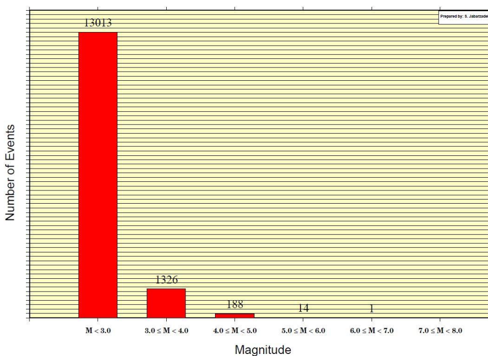
شکل ۱- فراوانی زمین‌لرزه‌های کشور بر اساس بزرگی در سال ۱۳۹۷
