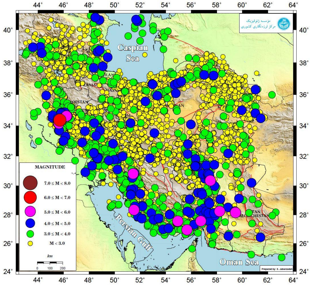
شکل ۲- نقشه رومرکز زمین لرزه‌های کشور در سال ۱۳۹۷
